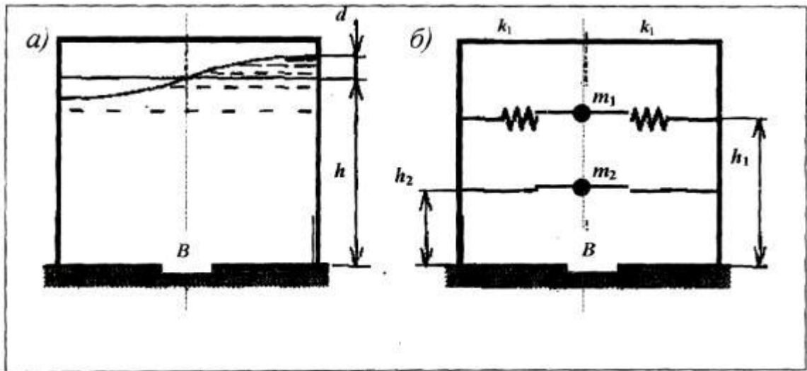
Рис.П.5.1. Моделирование резервуара с жидкостью:
