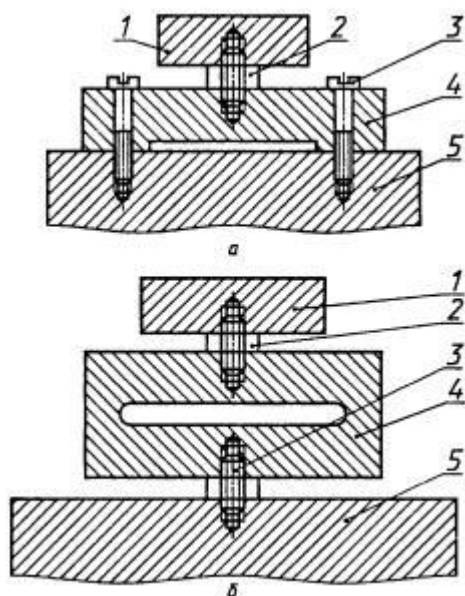
a - крепление балки к столу стенда в двух точках; б - крепление балки к столу стенда в одной точке 1 - приспособление для испытания изделий; 2, 3 - резьбовые шпильки; 4 - резонансная балка; 5 - стол вибрационного стенда
